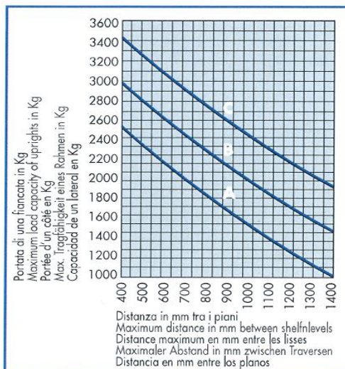
PORTATE DELLE FIANCATE MITO-EURO (SPALLA CONTROVENTATA)
